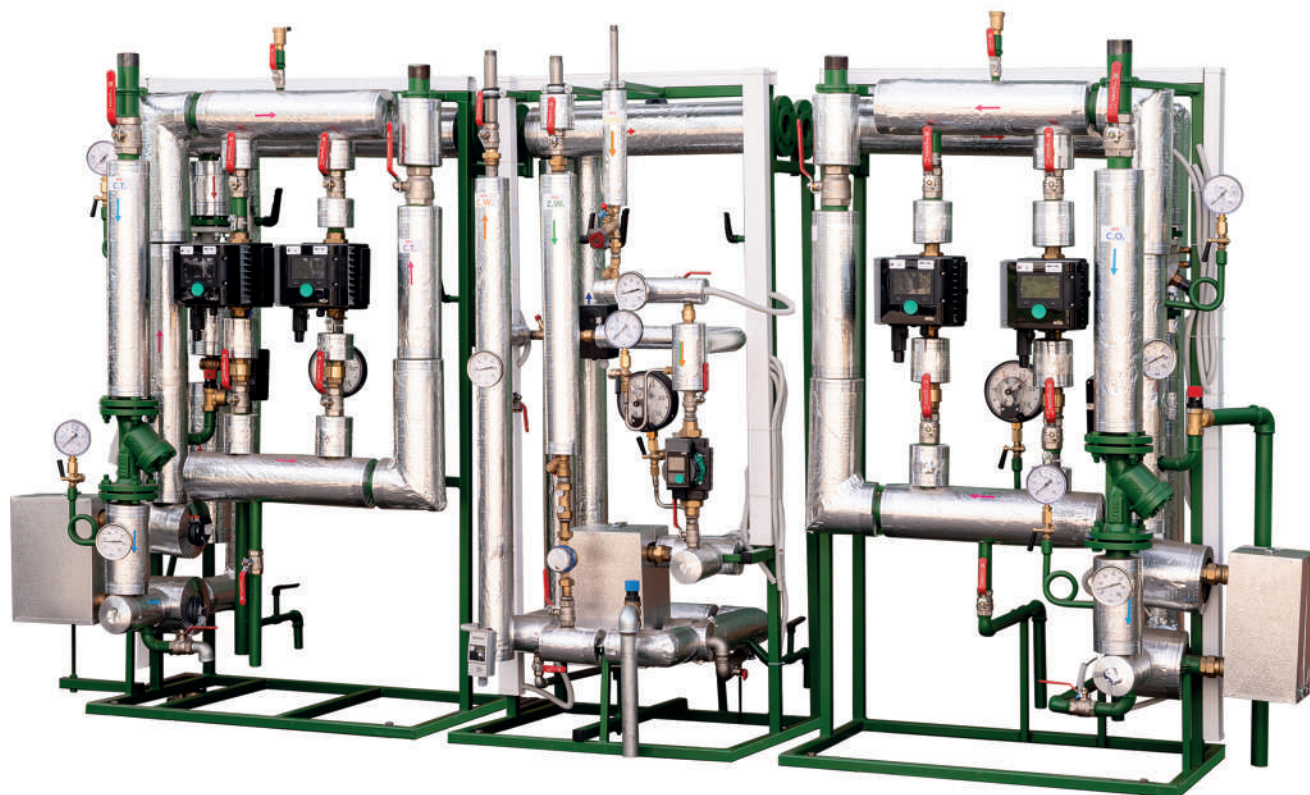
Węzeł 3-funkcyjny c.o., c.w.u. i c.t. dla budynku w Warszawie
